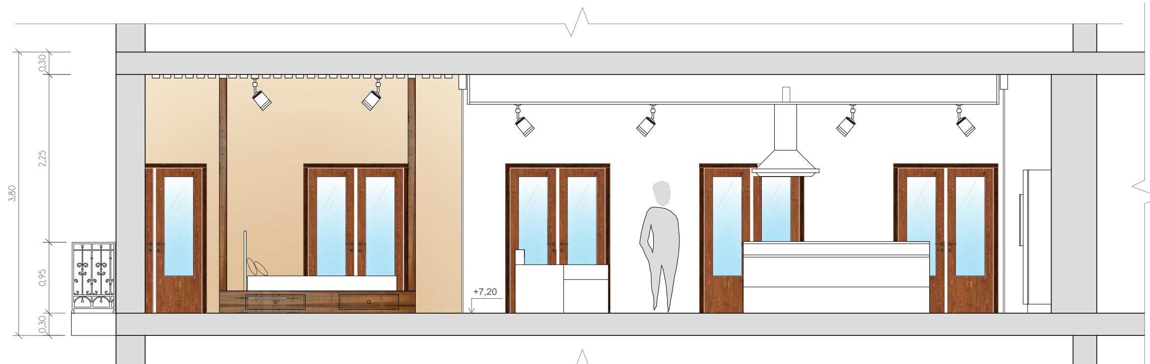
SECCIÓN A-A' Escala 1:50
